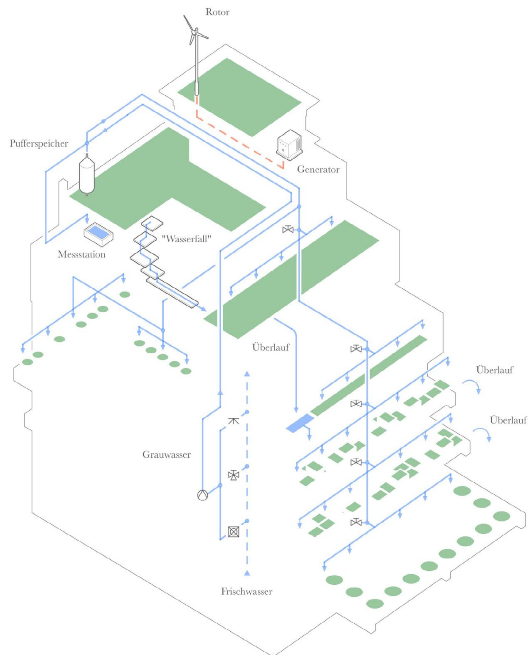
Axonometrie Wasser &-Energiekreislauf
