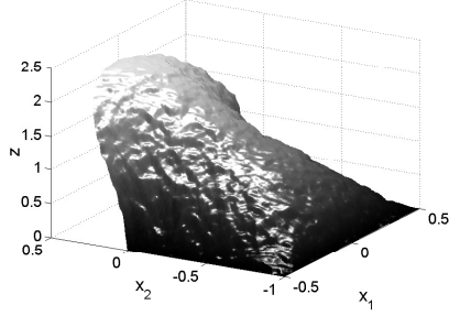
(a) Standard FEM. 10^6 DOF (finescale).
