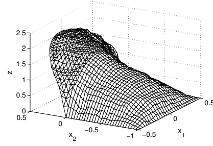
(d) FE-HMM with N_{micro} = 16 , \delta = 1.5 \cdot 10^{-2} . 1100 DOF (for macro mesh).
