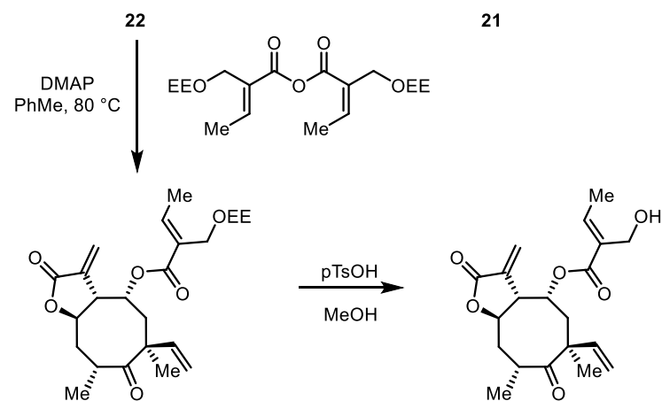
(±)-Jujuyane Org. Lett. 2021 , 23, 4651
