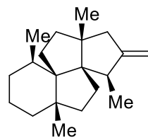
(+)-waihoensene
