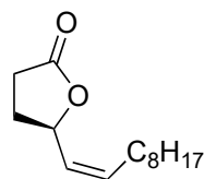
Japonilure
