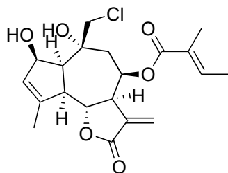
Eupalinilide E (1)
