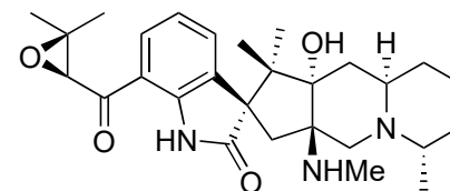
(+)-Citrinadin B
