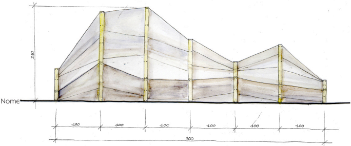
Élévation 1:20
