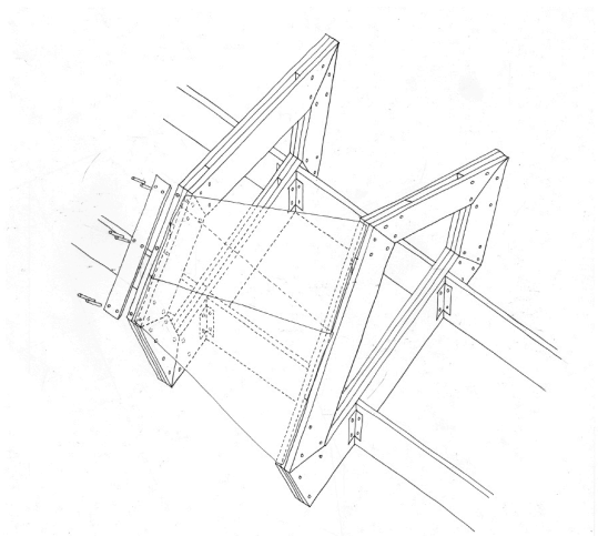
Axonométrie constructive partielle 1:10
