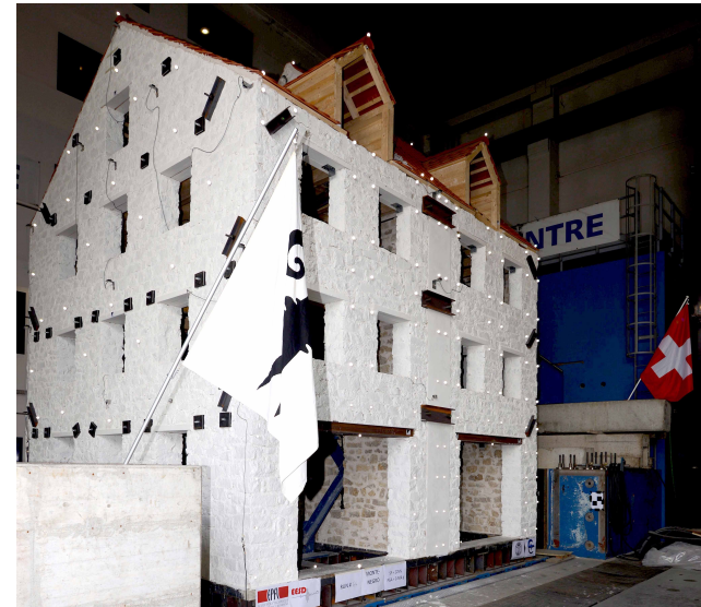
Rütteltischversuch mit zwei Basler Altstadt Häusern in Pavia
