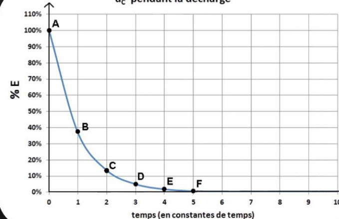
u_c pendant la décharge
